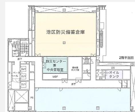
防災備蓄倉庫の設置状況(2階平面図)
